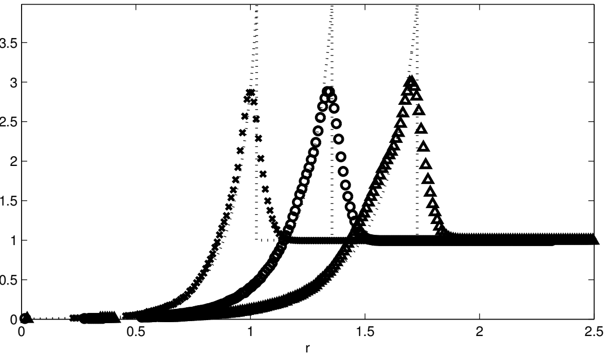
Density Sedov blast
